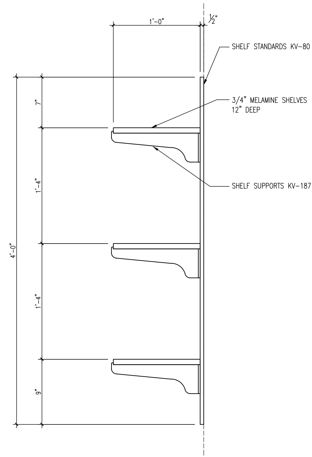
1 SECTION SD-9 SCALE: 1-1/2" = 1'-0"
