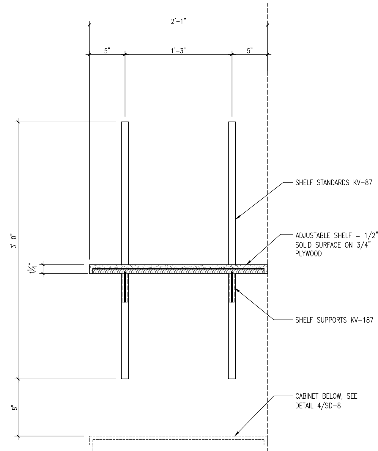
2 SECTION SD-9 SCALE: 1-1/2" = 1'-0"
