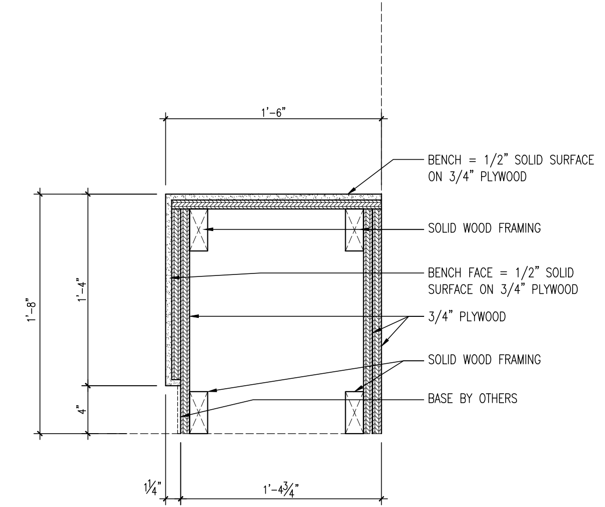
4 SECTION SD-9 SCALE: 1-1/2" = 1'-0"
