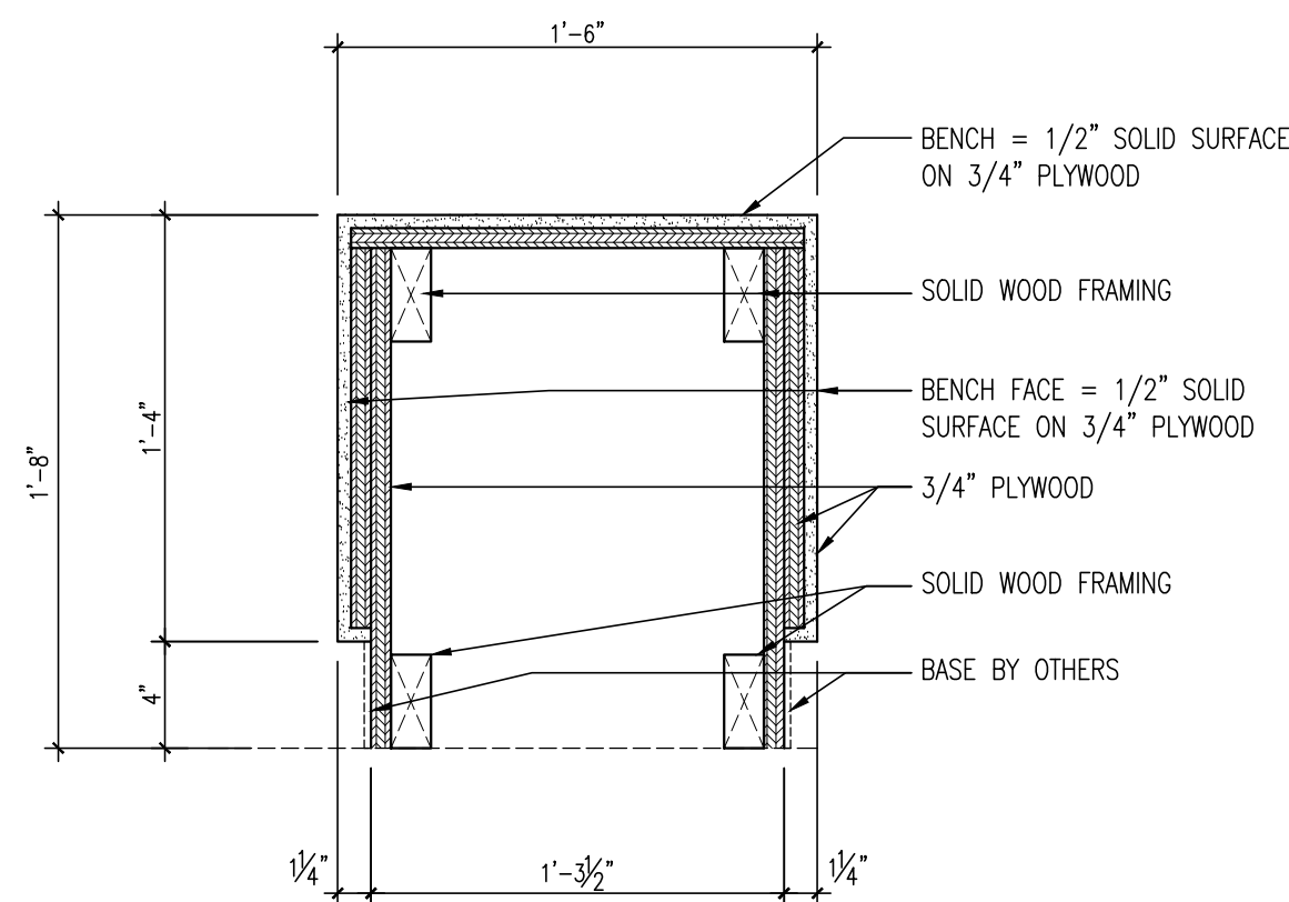
5 SECTION SD-9 SCALE: 1-1/2" = 1'-0"
